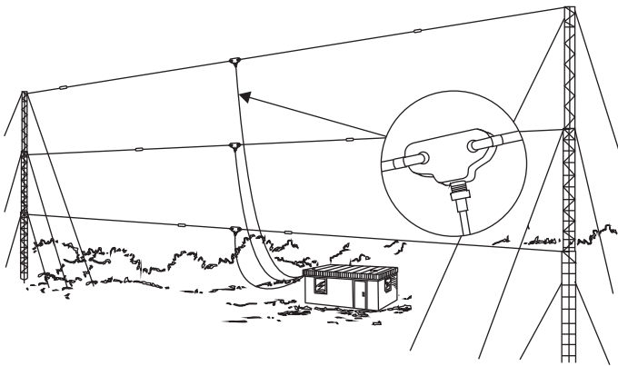
Varios dipolos unifilares de frecuencia única colocados entre dos torres.
