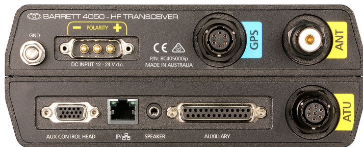
Barrett 4050 SDR Panneau arrière
