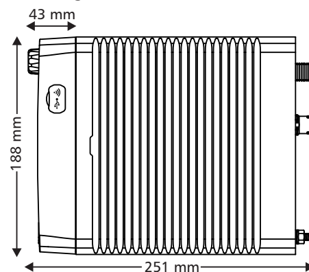
4050 Configuration de la station de base Poids 2.55 kg
