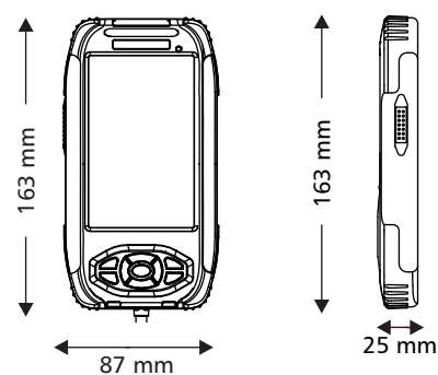
4050 contrôle combine Poids 0.28 kg
